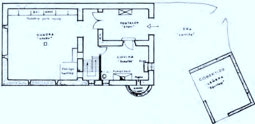
Jaureguibarria. — Planta baja.
