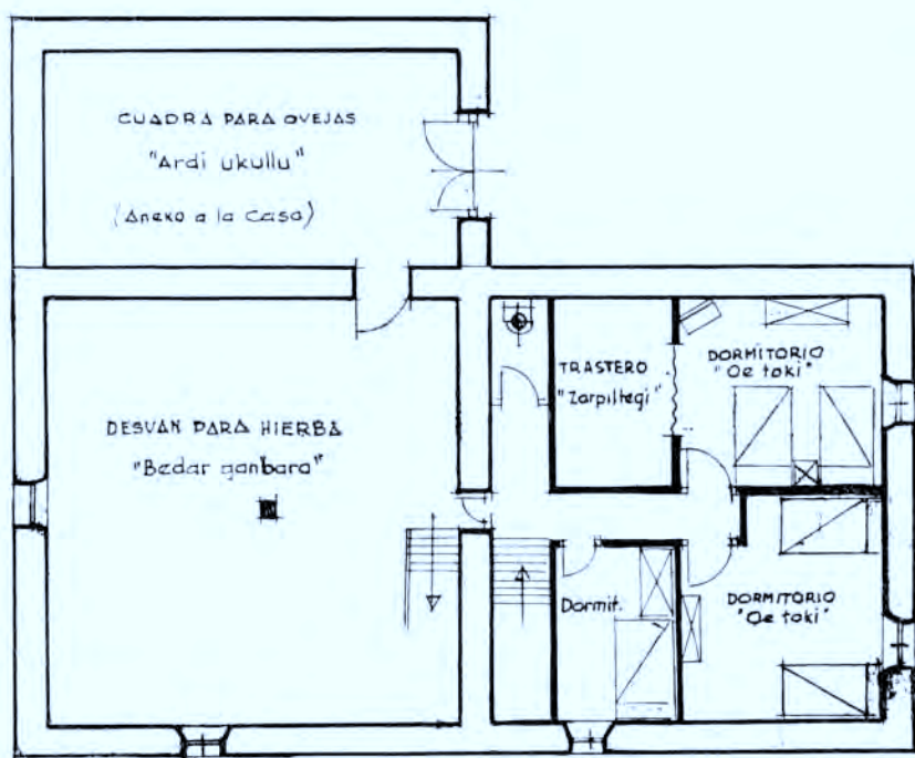
Jaureguibarria. — Segunda planta.
