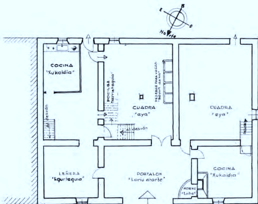
Casa grande de «ORTUZAR». — Planta baja.
