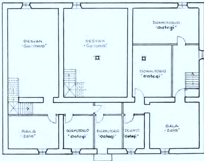
Casa grande de «ORTUZAR». — Planta piso.
